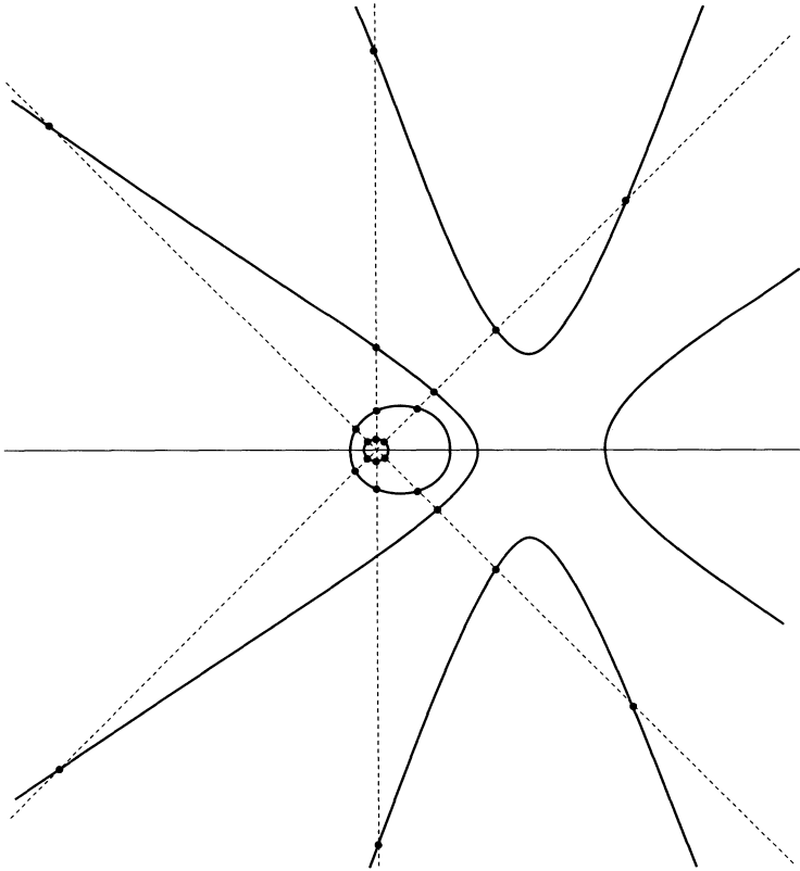
Figure 1 (cf. [P2]). La courbe \Delta_f = 0 où f(t) = \tilde{A}(t)/\tilde{E}(t) , avec \deg(\tilde{A}) = 7 et \deg(\tilde{E}) = 2 , rencontrant les b - 1 droites \Delta_{t^b}(x, y) = 0 en (b - 1)(\bar{a} + \bar{e} - 1) points à coordonnées réelles (on a ici \bar{a} = 7 , b = 4 et \bar{e} = 2 ).
