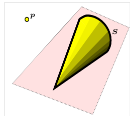
Base locus scheme \mathcal{B}(\mathcal{J}_{15}^5)
