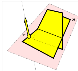
Base locus scheme \mathcal{B}(\mathcal{J}_6^5)
